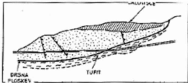
Shematski prerez plazu (vir: RŽV)
