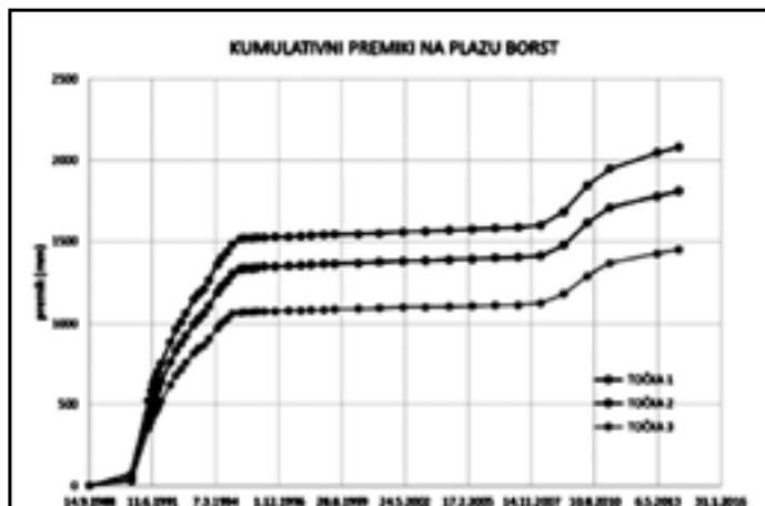
Premiki točk odlagališča hidrometalurške jalovine Boršt (vir: RŽV)
