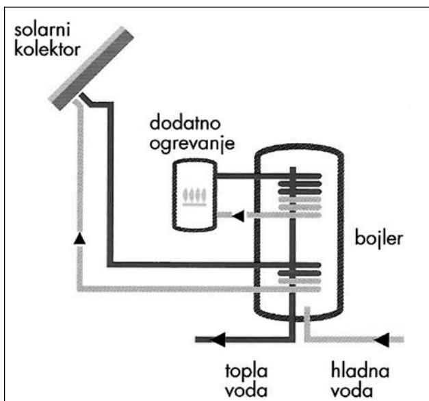
Bivalenten način gretja sanitarne vode s sprejemnikom sončne energije ali z drugim virom gretja, npr. prek kotla za centralno ogrevanje, z dodatnim plinskim ogrevanjem.
